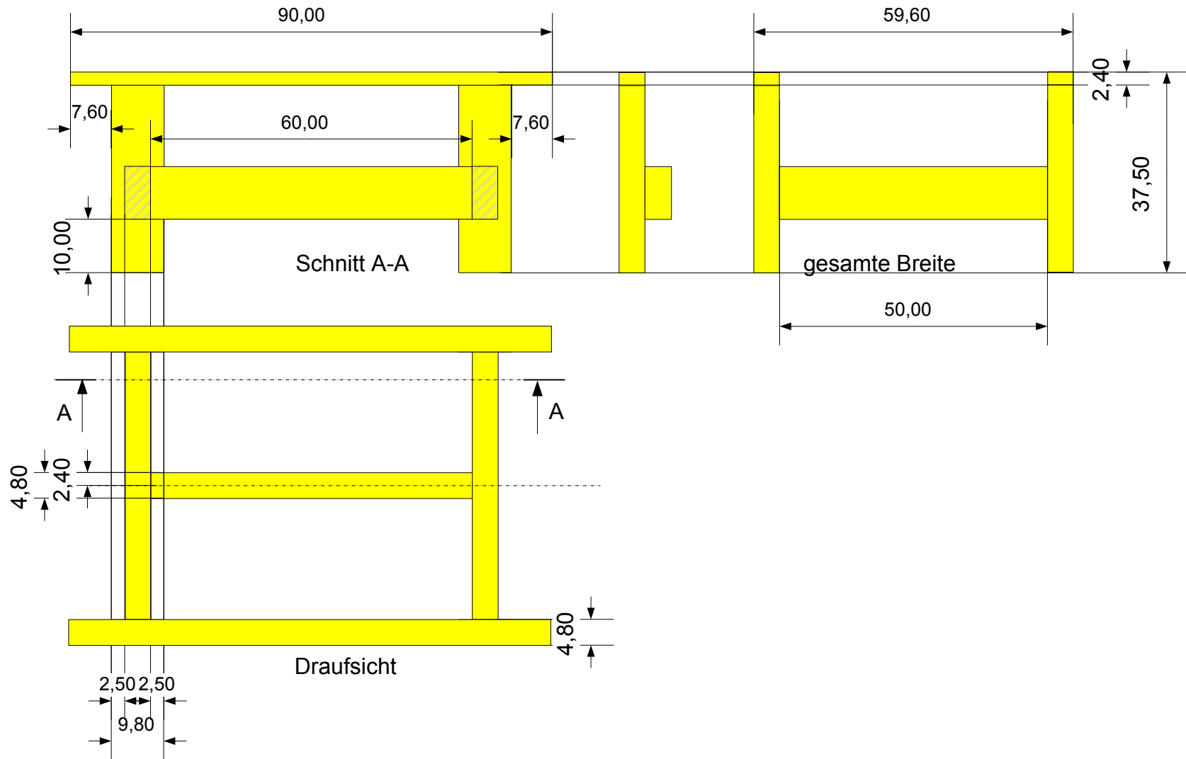
Couchtisch für Tischplatte 80 x 120 cm Aufriß pm – 2008-04-10 Maße: cm
